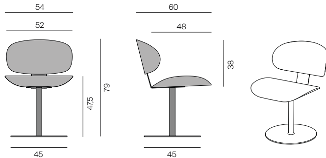
LUZ Drehstuhl, ohne Armlehne LUZ Swivel chair, without armrest
